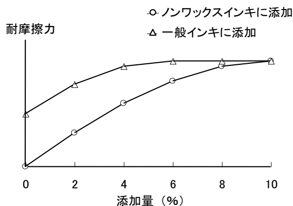
コンパウンドの添加量と耐摩擦性
